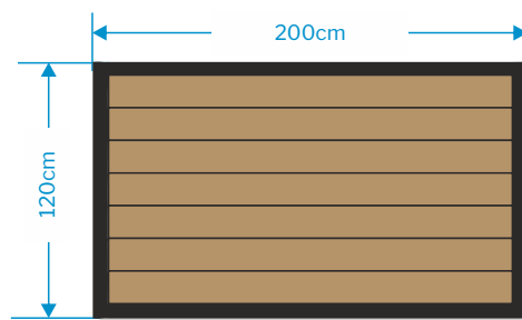
Przęsło ogrodzeniowe
