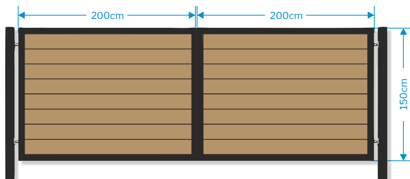
Brama rozwierna dwuskrzydłowa
