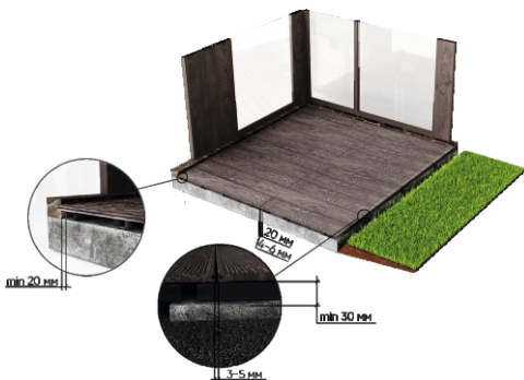
Rys. 5. Układanie deski na konstrukcji metalowej.
