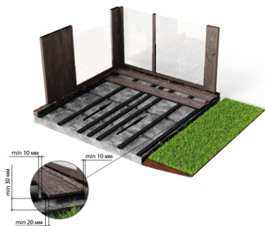
Rys. 3. Układanie deski na legarze.
