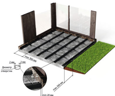
Rys. 4. Układanie i mocowanie deski (patrz tab. 1).
