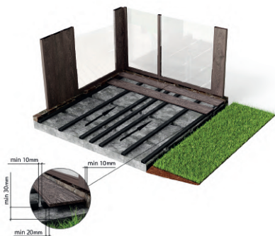
Rys. 3. Układanie deski na legarze.
