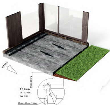
Rys. 1. Układanie legara na podłożu betonowym.
