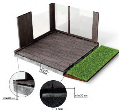
Rys. 5. Układanie deski na konstrukcji metalowej.
