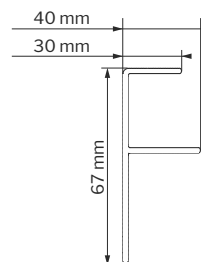
Przekroje
